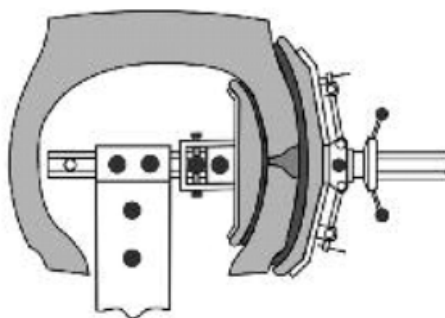
Рисунок 3.7 – Ремонт боковини
