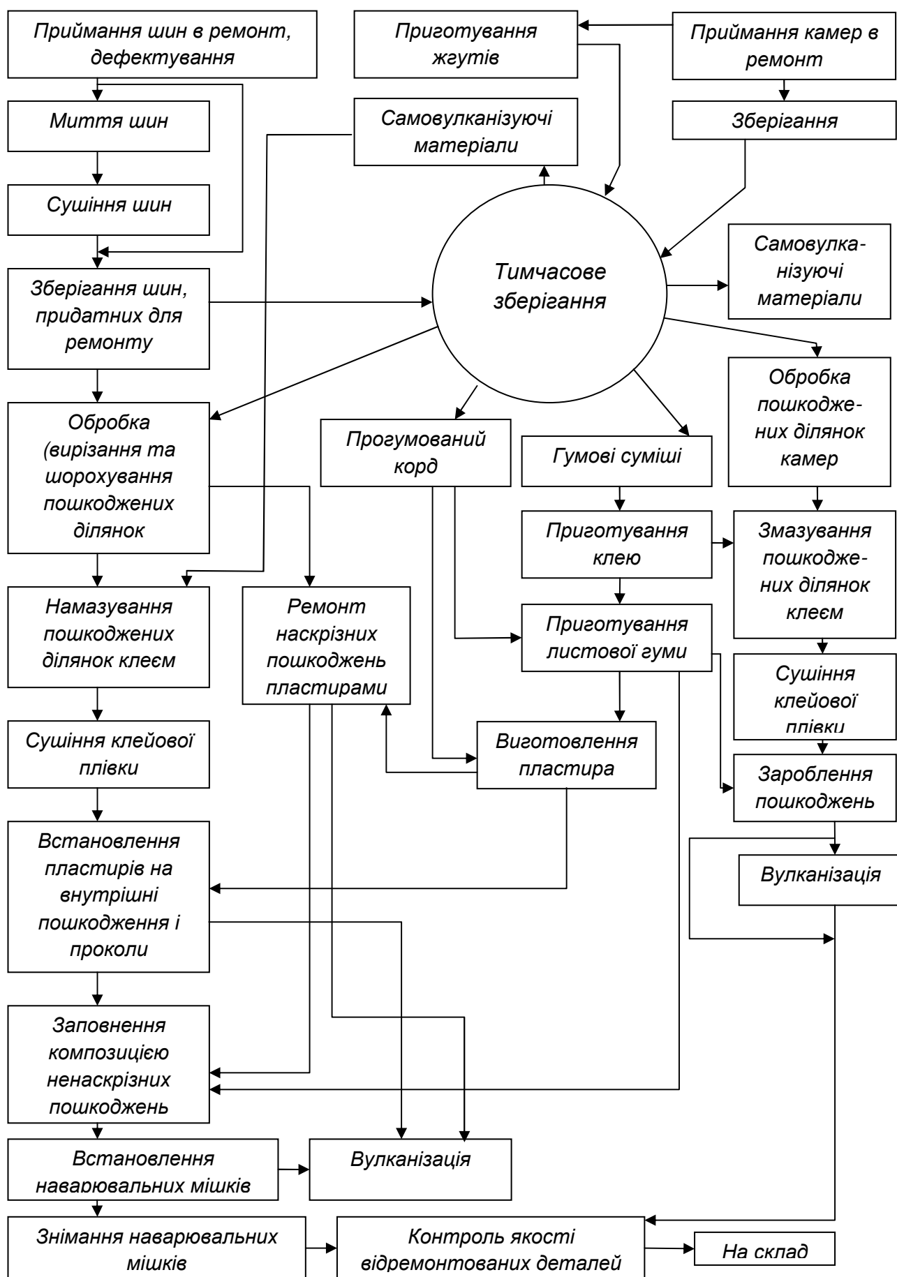
Рисунок 2.1 – Удосконалена схема робіт шиноремонтної дільниці
