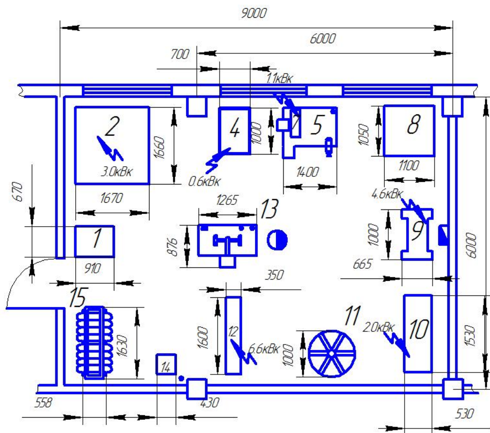
Рисунок 1.6 – Типовий план шиноремонтної дільниці: 1 – скриня для інструментів; 2 – шиномонтажний верстат; 3 – вентиляція; 4 – верстат для рихтування дисків; 5 – слюсарний верстат; 7 – шліфувальна машина ручна; 8 – мийна ванна; 9 – шліфувальний верстат; 10 – вулканізатор; 11 – оглядовий стенд; 12 – клітка для накачування; 13 – шиномонтажний верстат для шин великих розмірів; 14 – криця для відходів; 15 – стелаж для зберігання коліс.
