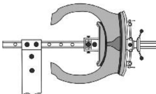
Рисунок 3.5 – Ескіз монтажу шини на вулканізатор
