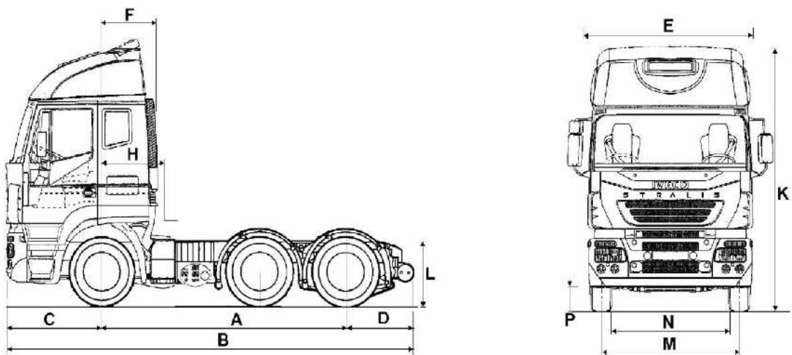
Рисунок 3.4 – Загальний вигляд автомобіля тягача Iveco-Stralis
