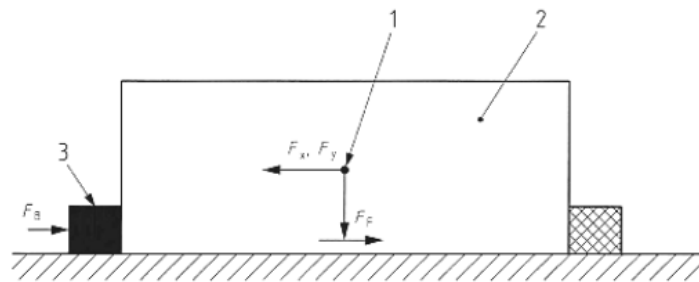
Рисунок 3.10 – Кріплення вантажу блокуванням
