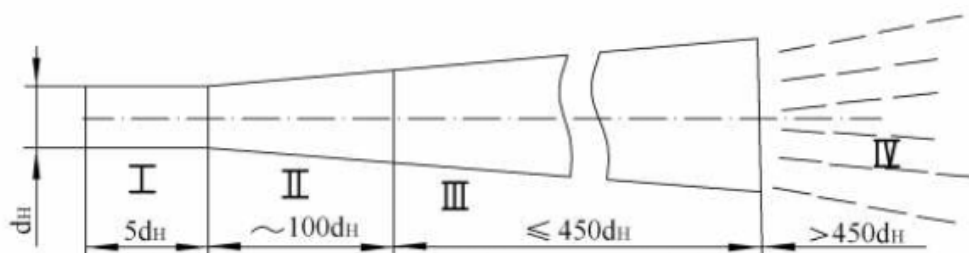
Рисунок 2.5 – Схема вільного струменя
