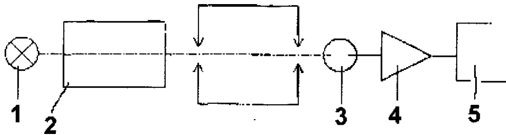
Рис. 2.4. Функціональна схема атомно-абсорбційного спектрофотометра:
